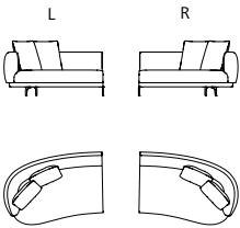
850-20 A2 W 171 D 124 H 71/73 SH 42/44 SD 79
