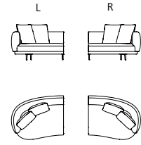
850-15 A2 W 141 D 115 H 71/73 SH 42/44 SD 79
