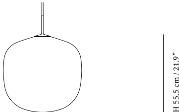
Rime Pendant Lamp — Ø 45 cm / 17.7" Ø 45 cm / 17.7"
