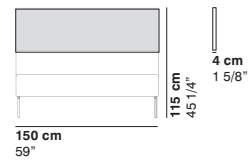
cod. 1213 / back panel 150 h. 115
